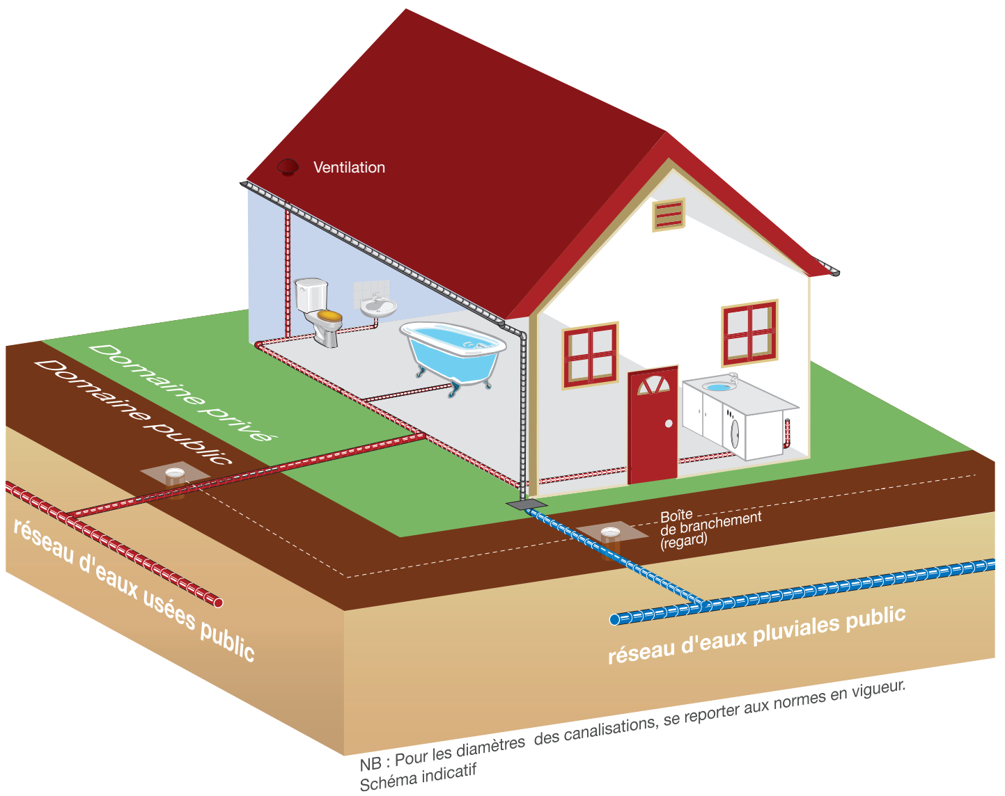
Schéma de principe du branchement d'une habitation
